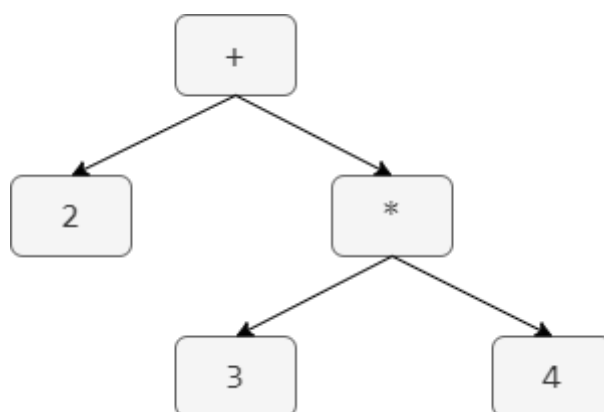
Рисунок 1.3. AST выражения 2 + 3 * 4
